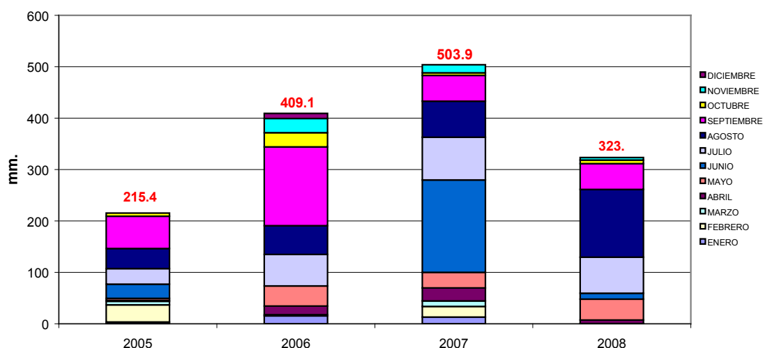
PRECIPITACIÓN MEDIA MENSUAL ACUMULADA EN SAN LUIS POTOSÍ, DURANTE LOS AÑOS 2005,2006,2007 y 2008.
