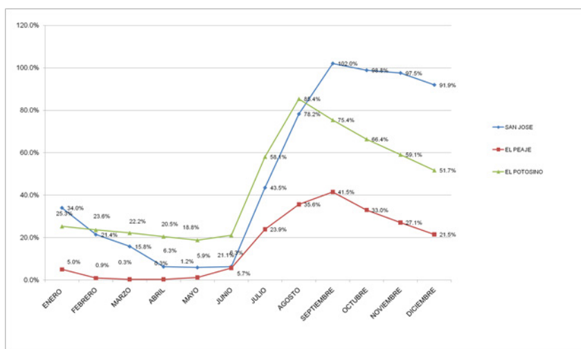
Porcentaje de Almacenamiento de Presas
